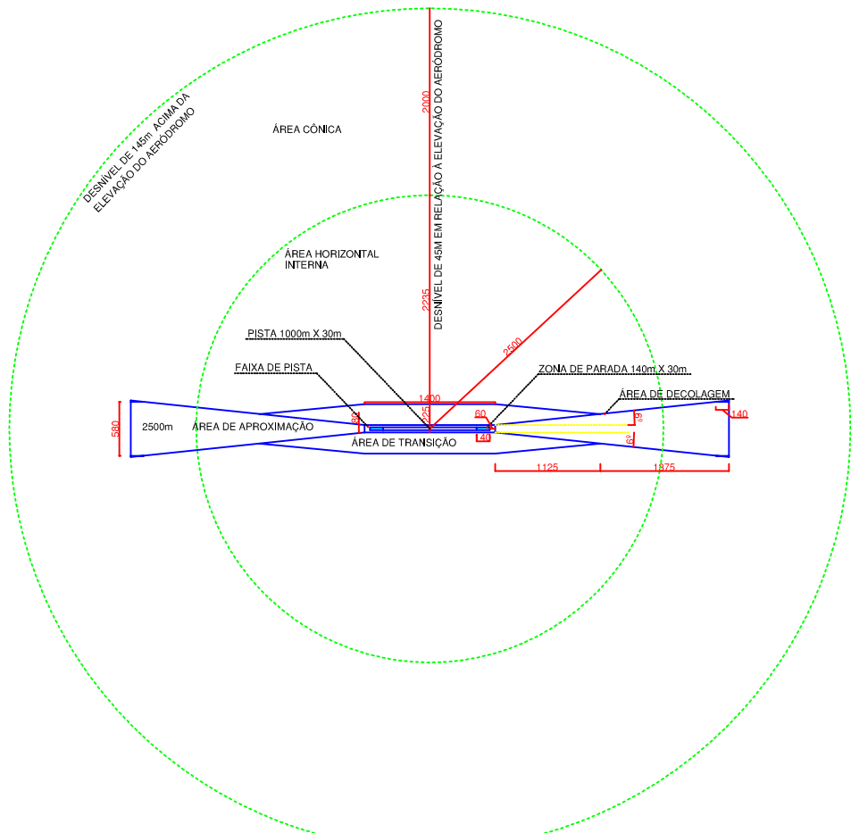
Plano Básico de Zona de Proteção de Aeródromo (portaria nº 1141/GM5 de 18/12/87) Classe VFR - Código de Pista 2
